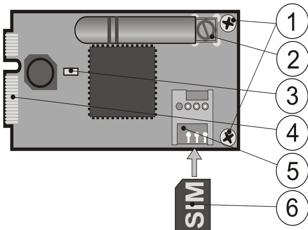
Rys. 1: Komunikator JA-194Y
